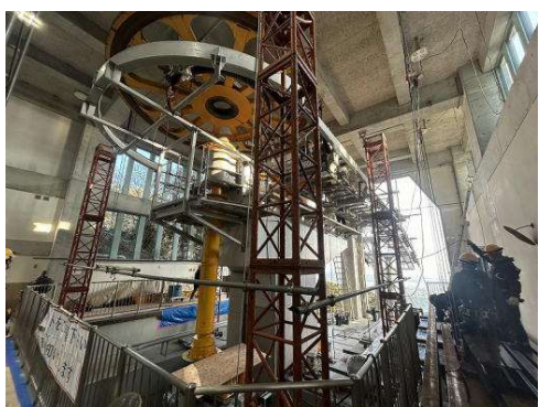
原動滑車整備
