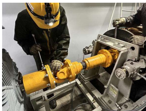
ユニバーサルジョイント更新
